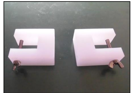
3) MPM用ストッパー(厚み約28mm) (左右セット・ネジ付き) 部品番号: 3946 ¥6,800
