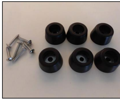
5) ゴム足6個1組(ネジ付き) 部品番号: 3927 ¥3,600
